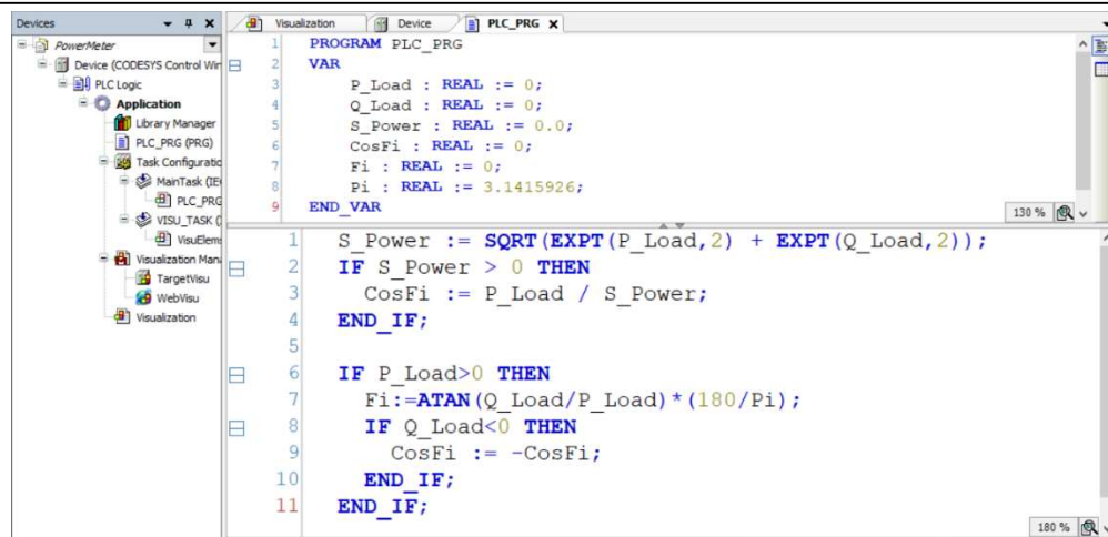
Рисунок 1 — Програмний код в середовищі CODESYS для розрахунку повної потужності та коефіцієнта потужності \cos \varphi .
