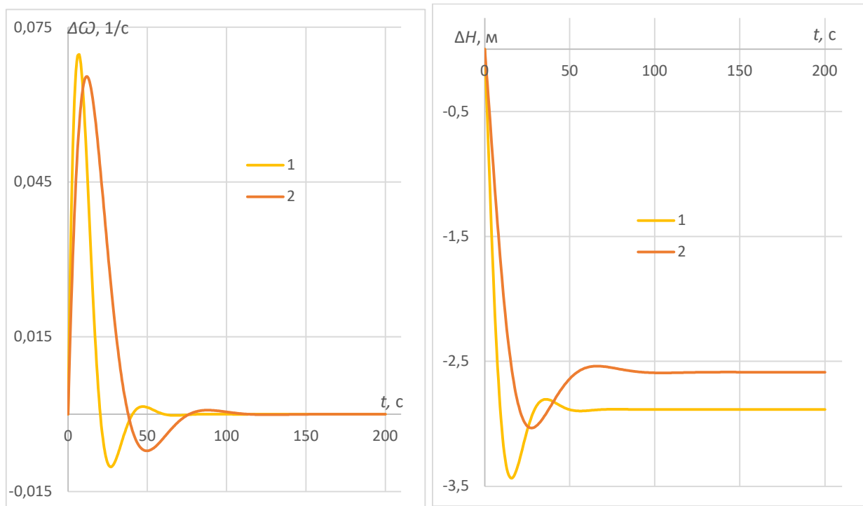
Рисунок 1 — Залежності \Delta\omega, 1/c і \Delta H, m від часу t, c
