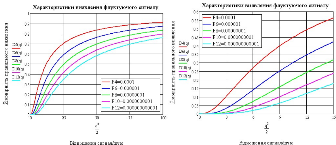
Рисунок 1 — Характеристики виявлення D = f(F, q) для флуктуючого сигналу з випадковою фазою
