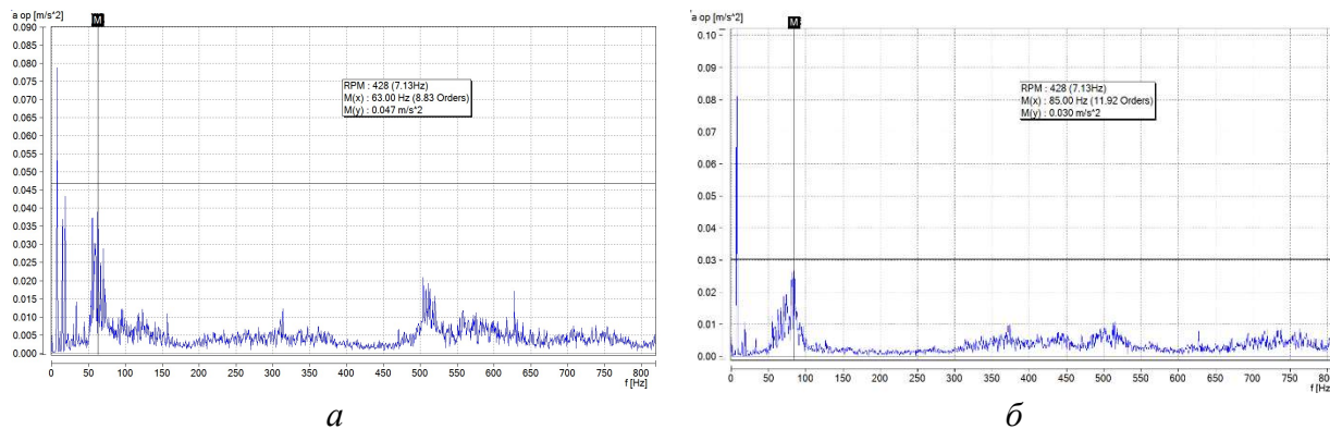
Рисунок 4 — Фрагмент спектру віброприскорення зі сторони вхідного валу:
