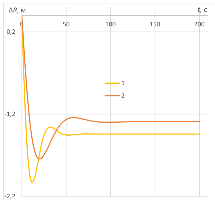
Рисунок 2 — Залежності \Delta R, m від часу t, c
