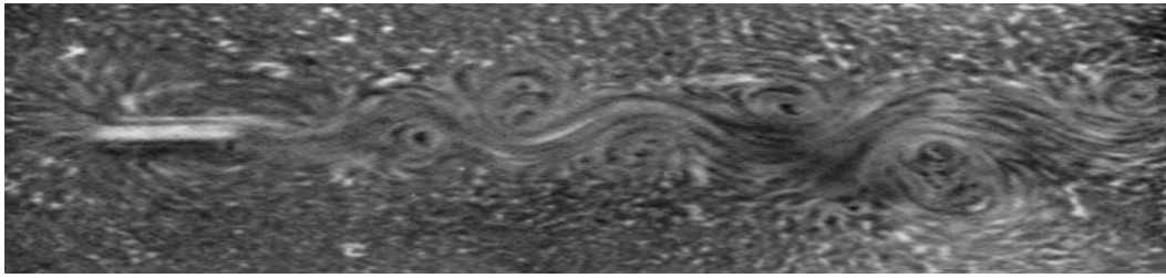
Рисунок 2 — Вихорова доріжка в сліді колового циліндра: а — розрахунок (блок 3) Re = 19\,300 ; б — експеримент Re = 19\,300 [9,10]
