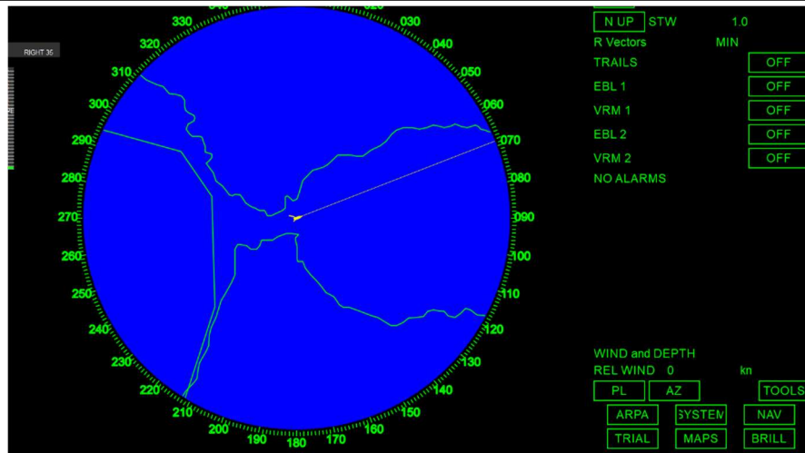
Рисунок 3 — Відображення маршруту
